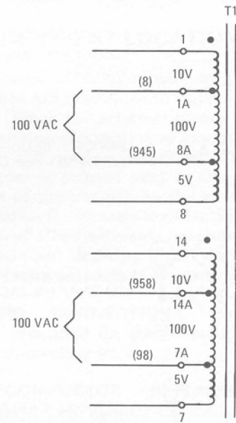
Option 003 Wiring
